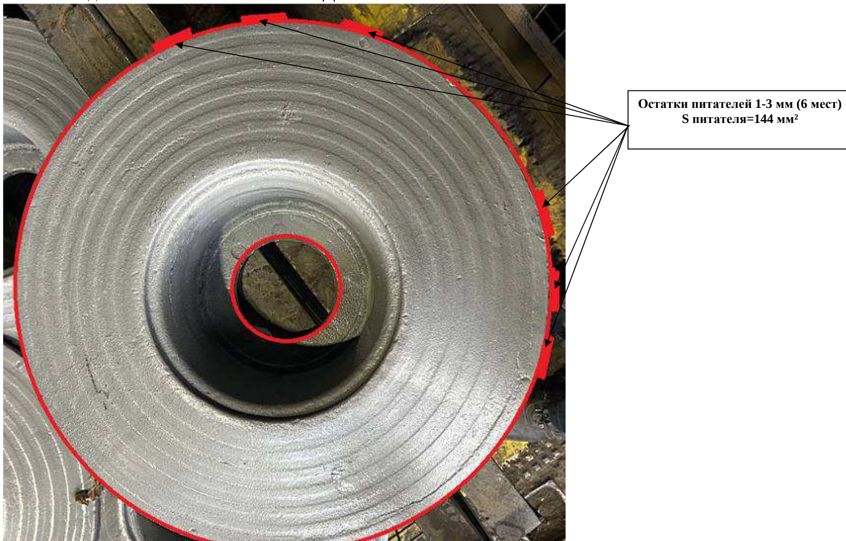
Рис.2 - Внешний вид отливки РСМ 10.01.15.102Г Диск
